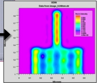
この図は、シルバコの Optolith と共に使用した場合のマルチフィンガー・テストパターン 1 の180°位相シフトを示しています。
