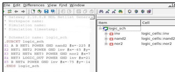
図3. ネットリスト・エディタ
