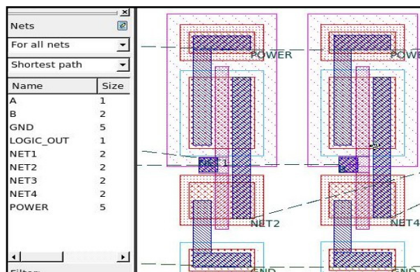
図4. ネット・フライトラインを示したレイアウト・インスタンス
