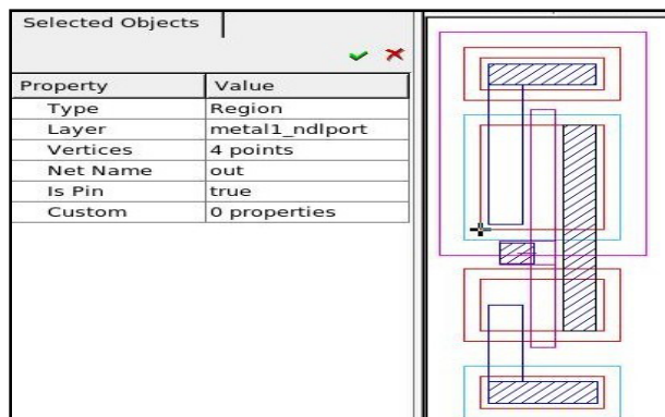
図2. インバータ・レイアウト・セル'out'ポートを表示したプロパティ・ウィンドウ
